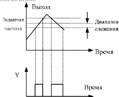
Рис.7-23 Сигнал при отклонении частоты.
