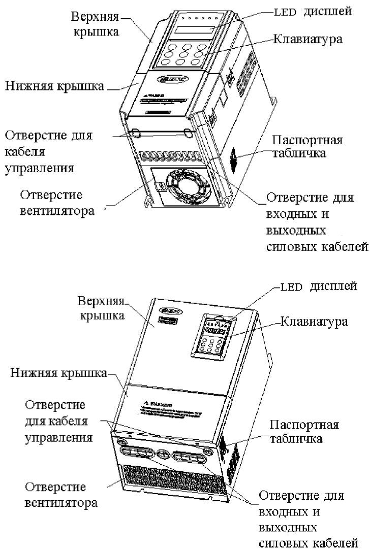
Рис.2-3 Внешний вид и наименование деталей EN600.
