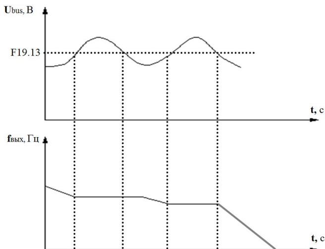
Рис. 7-46 Перенапряжение.
