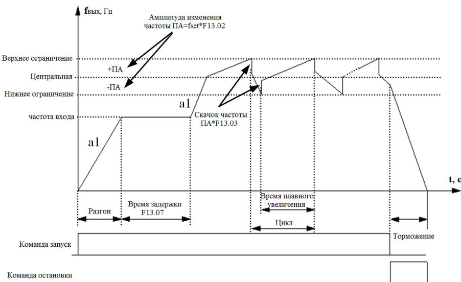
Рис.7-43 График работы в режиме плавающей частоты.
