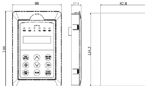
Рис. 2-8 Установочные размеры.
