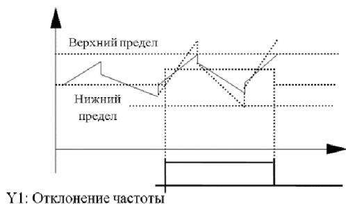
Рис.7-22 Отклонение частоты
