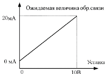
Рис.7-38 Соотношение задания и обратной связи.
