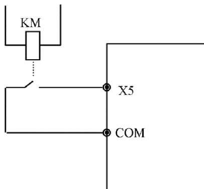
Рис. 7-15 Реализация подачи сигнала на дискретный вход.
