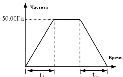
Рис. 7-1. Линейное ускор/торм
