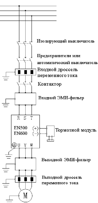
Рис.3-8 Типовое подключение преобразователя частоты.
