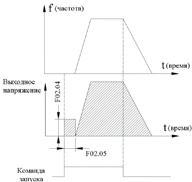
Рис. 7-4 Описание режима запуска 1.
