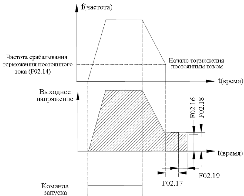
Рис. 7-5 Замедление и торможение постоянным током.
