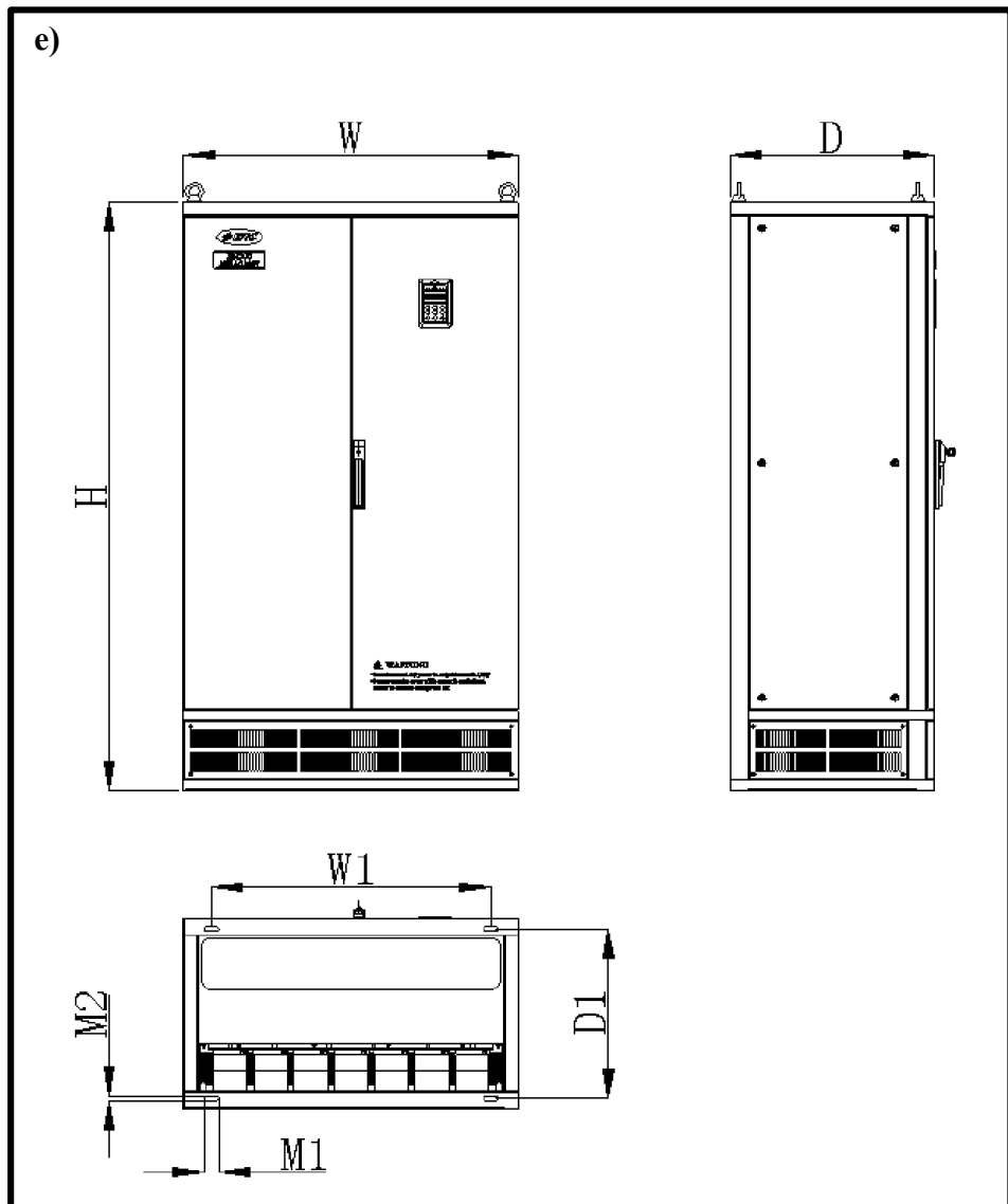
Рис.2-5 Внешние размеры
