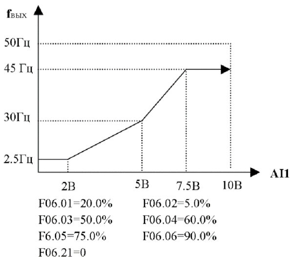
Рисунок 7-11 – Пример настройки зависимости кривой 1 входного сигнала на АП и реакции при снижении входного сигнала ниже минимума.
