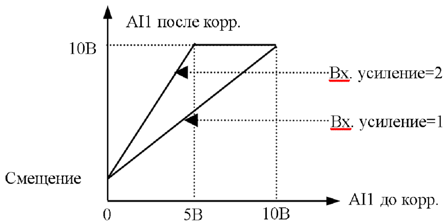
Рис. 7-12 Корректировка значения на входе АП1.
