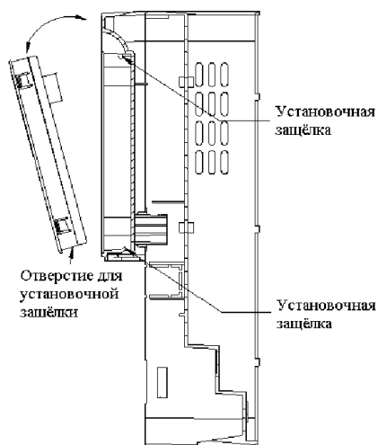
Рисунок 3-3 Установка пульта.
