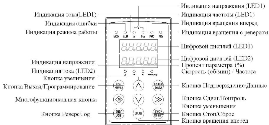
Рис.С-1 Расположение органов управления на панели EN-LED2.
