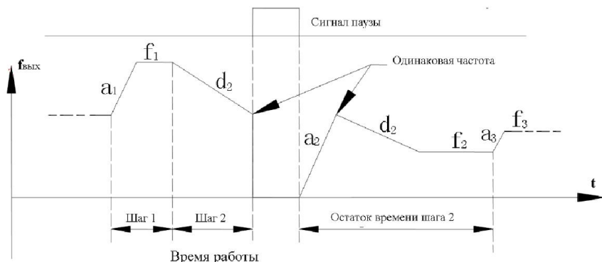
Рис.7-35 Режим 2 перезапуска ПЛК ( a_1 , a_2 , a_3 – время ускорения 1-ого ш, 2-ого, 3-его шагов, соответственно; d_2 – время торможения 1-ого шага; f_1 , f_2 , f_3 – частоты шагов).
