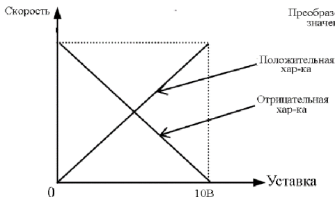
Рис. 7-40 Выходная характеристика.
