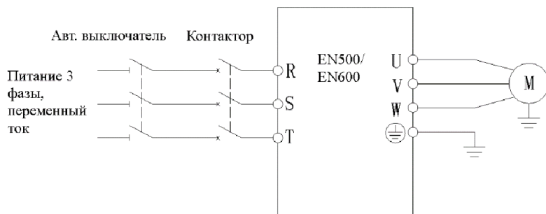
Рис.3-7 Простейшая схема подключения силовой части
