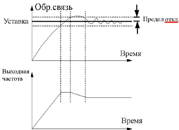
Рис.7-39 Предел отклонения.
