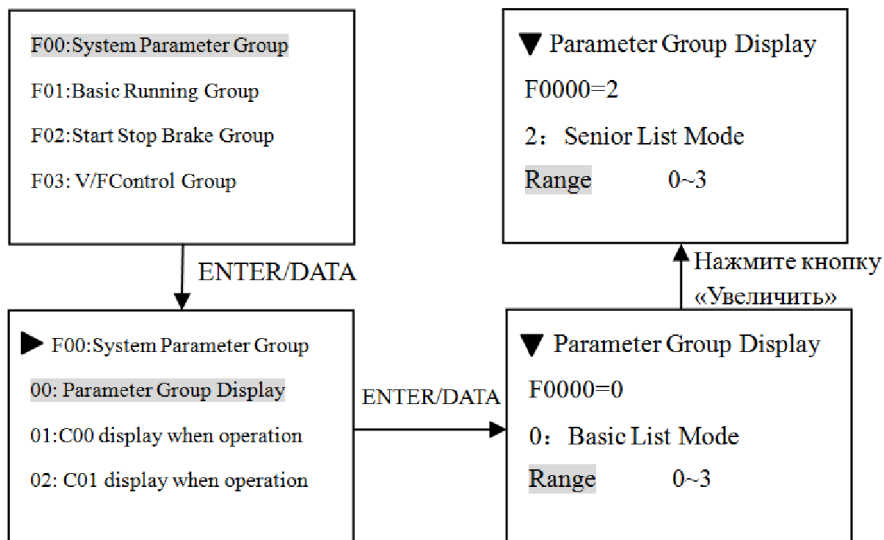
Рис.С-5 Пример управления в подменю.
