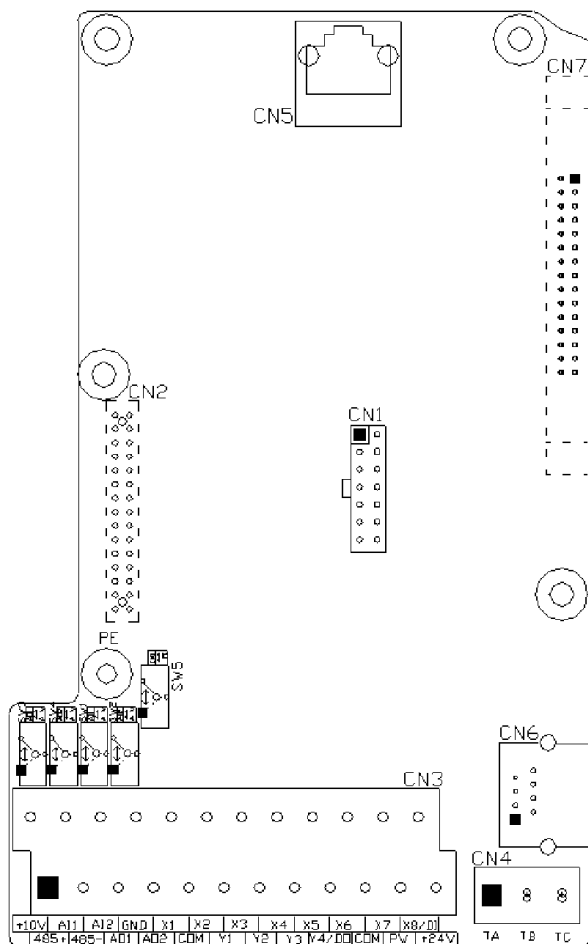
Рис 3-10 Управляющая плата (схематично)
