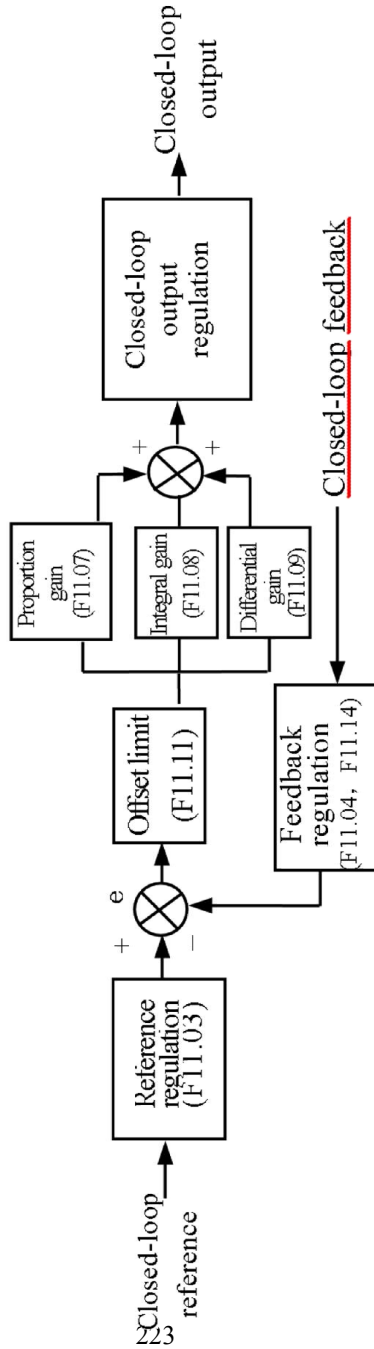
Рис.7-37 Принцип работы ПИД-регулятора.
